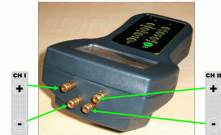
Méréselőkészítő
