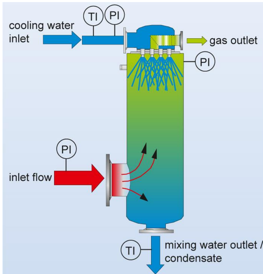
1. ábra A keverő kondenzátor kapcsolási sémája
